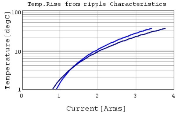
GRM219R71E105KA88 Temp.rise — 500kHz
